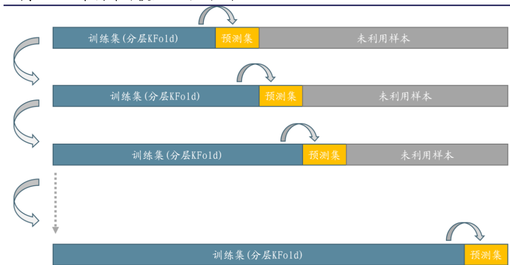
图表 4、决策树择时模型回测流程图
